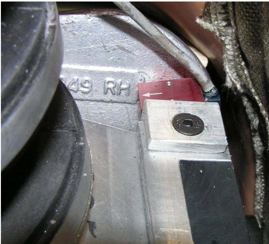
Bild 4, placering av T1-accelerometern i krockdockan
