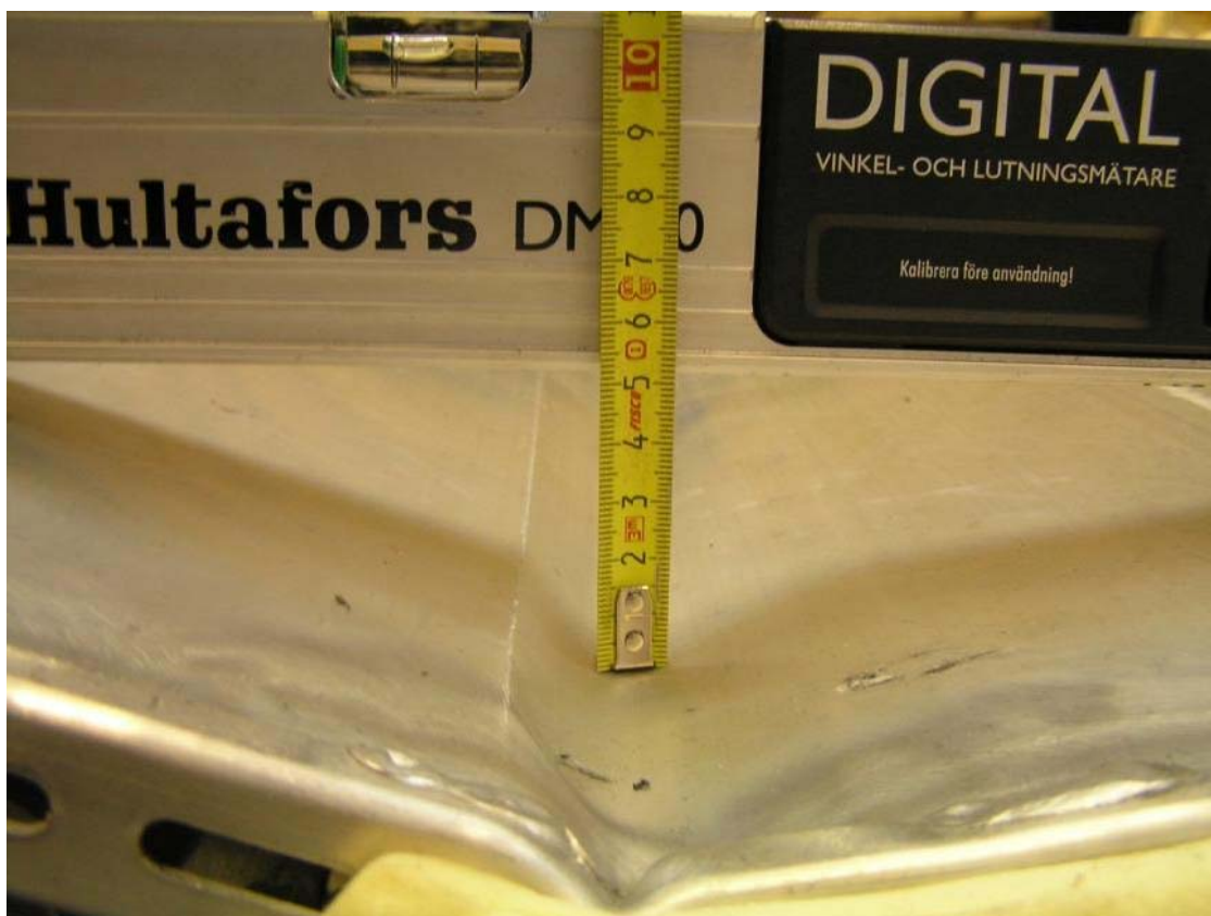
Bild 6, Mätning av den horisontella deformationen av sätesryggen
